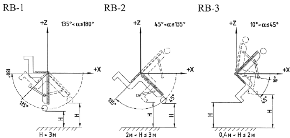
Рис. 1. Наклон пассажирских кресел вперед
