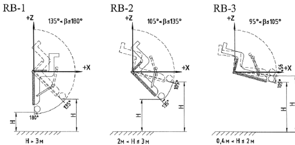
Рис. 2. Наклон пассажирских кресел назад
